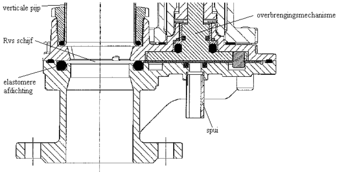
Principetekening 2.
