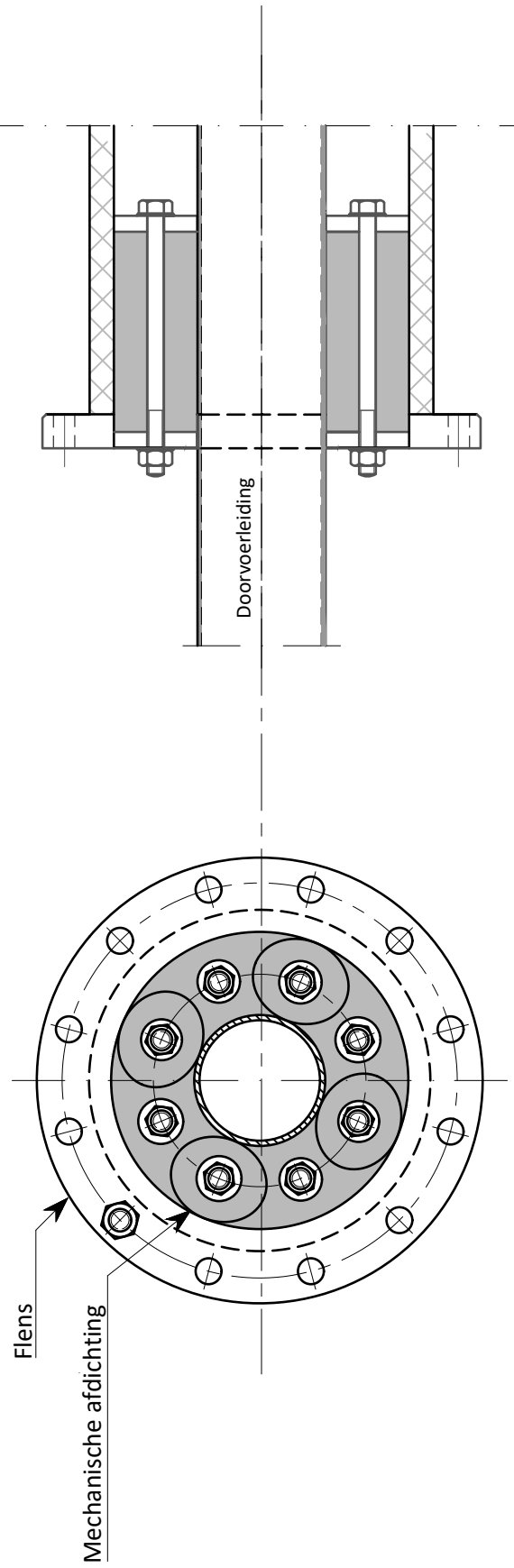
Snede C-D:
