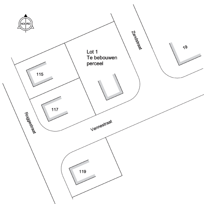
Voorbeeld inplantingsplan
