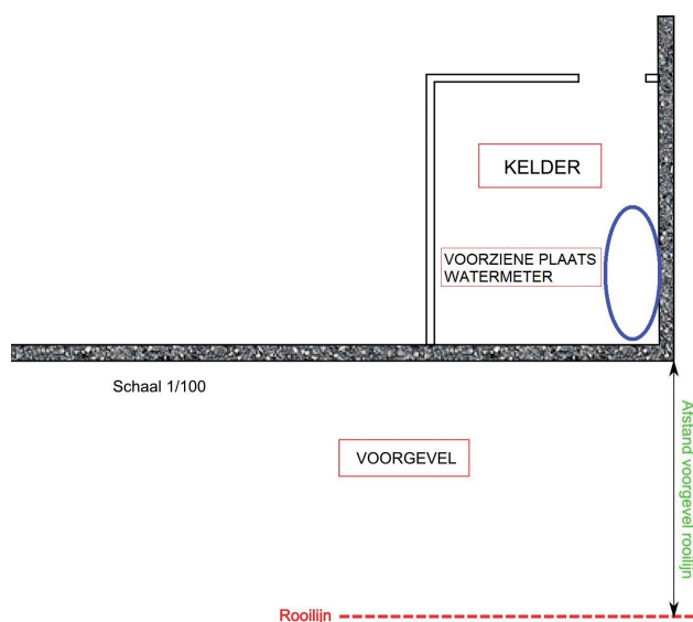
Voorbeeld plan met aanduiding gewenste plaats watermeter
